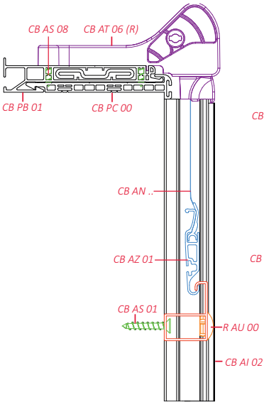
widok z boku A-A
