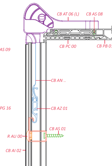
widok z boku B-B
