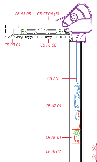
widok z boku A-A
